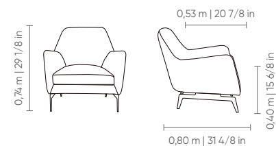
Pé Aço carbono
