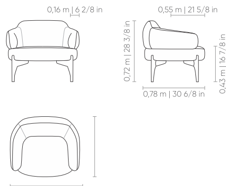
DIMENSÕES DIMENSIONS | DIMENSIONES
