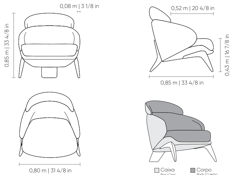
POLTRONA armchair | sillone
