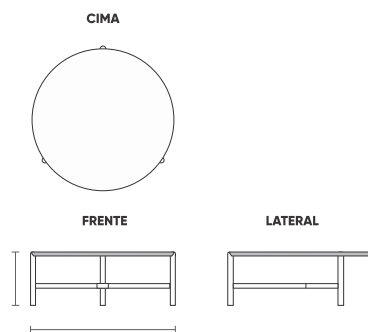
MESA REDONDA ALT 0,42 x 0,42 m 0,45 m 0,95 x 0,95 m 0,34 m
